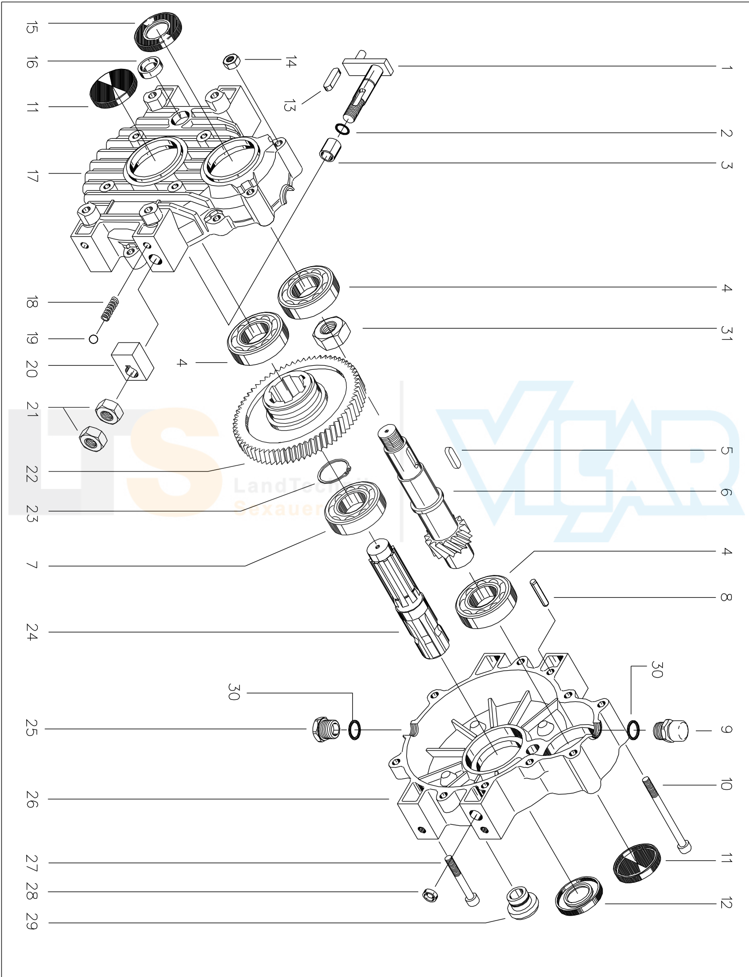
Getriebe / Gearbox TU600 (Cod. 500011)
