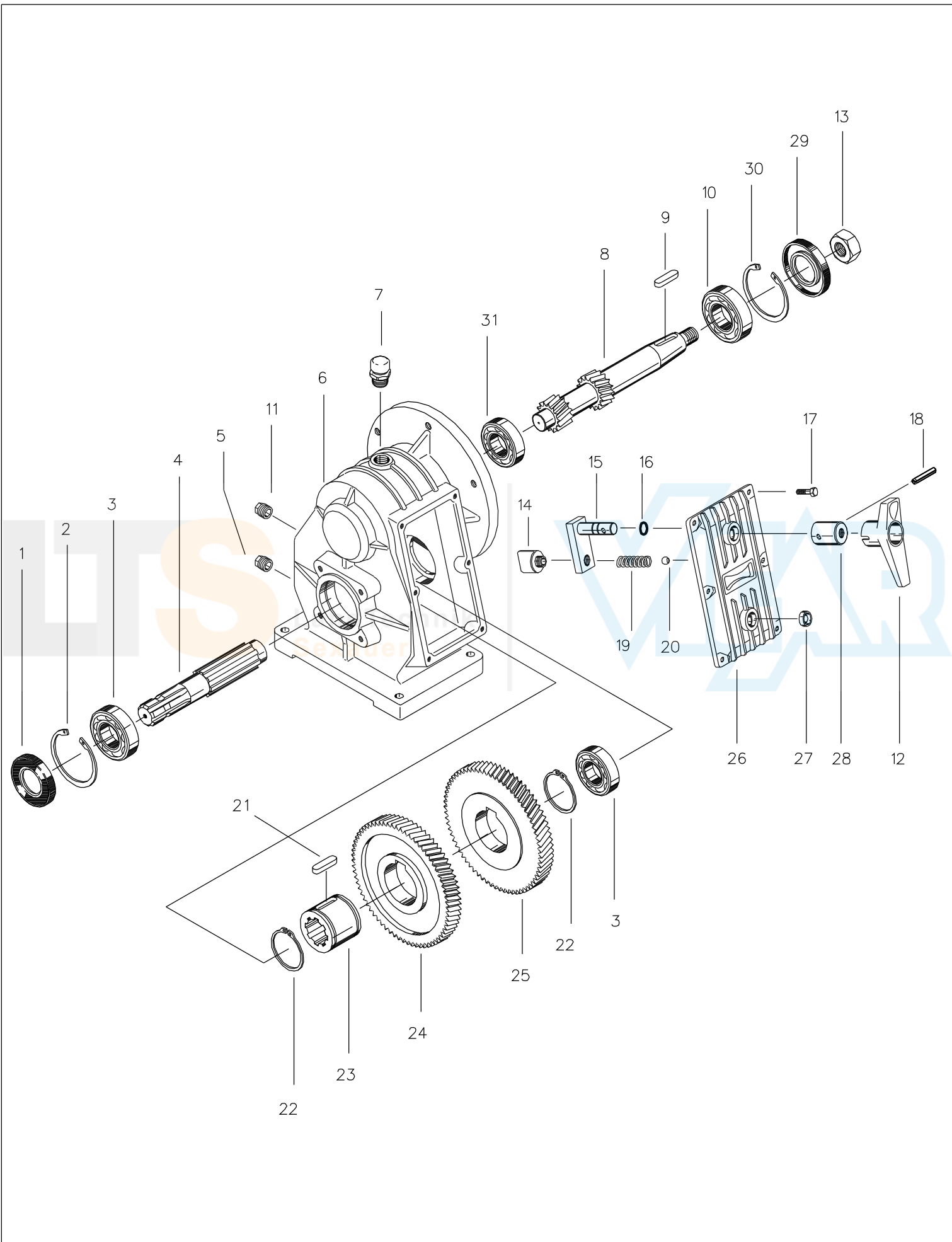
Getriebe / Gearbox 450, 456 (Cod. 500018)
